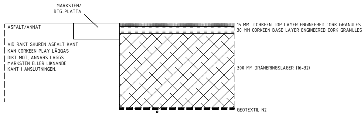
ANSLUTNING CORKEEN PLAY MOT HÅRDGJORDA YTOR TYP ASFALT, BETONGMARKSTEN M.M. SKALA 1:10
