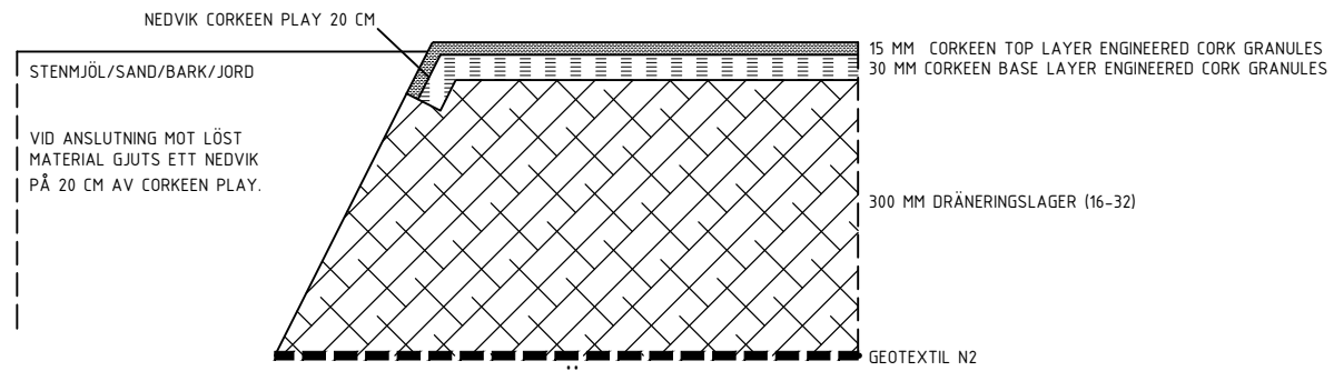
ANSLUTNING CORKEEN PLAY MOT LÖSA MATERIAL TYP STENMJÖL, SAND, BARK M.M. SKALA 1:10
