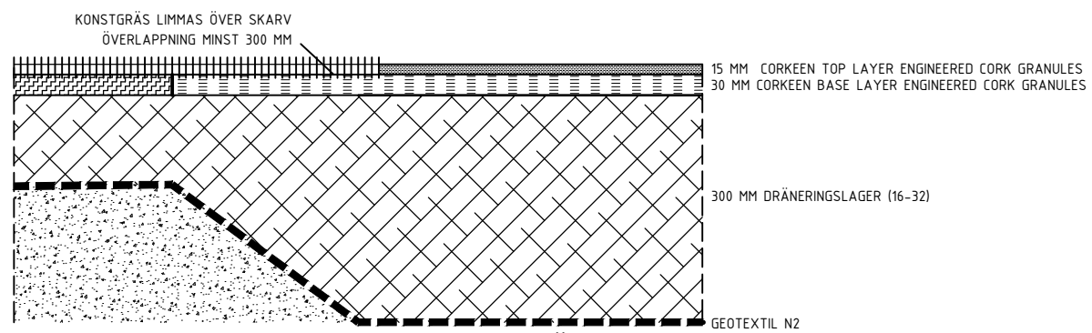
DOLD KANT CORKEEN PLAY MOT KONSTGRÄS SKALA 1:10
