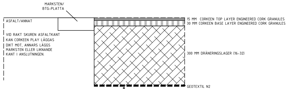
ANSLUTNING CORKEEN PLAY MOT HÄRDGJORDA YTOR TYP ASFALT, BETONGMARKSTEN M.M. SKALA 1:10
