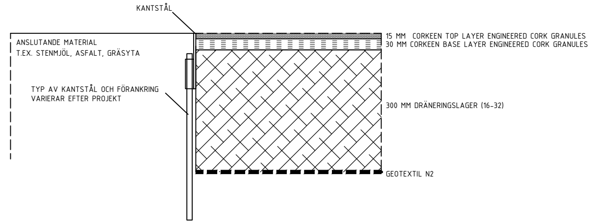
ANSLUTNING CORKEEN PLAY MOT KANTSTÅL SKALA 1:10
